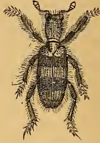
Fig. 86. TRICHODES APIARIUS.
